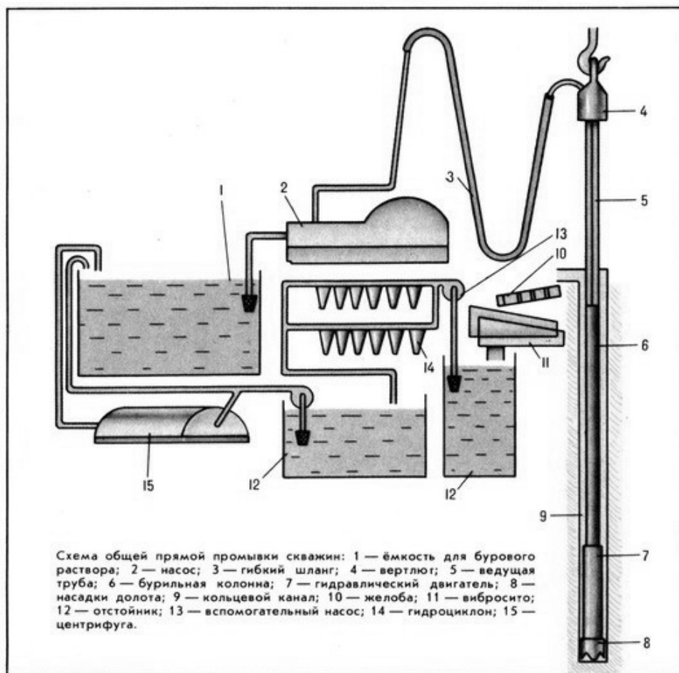
Рисунок 1. Схема общей прямой промывки скважин
