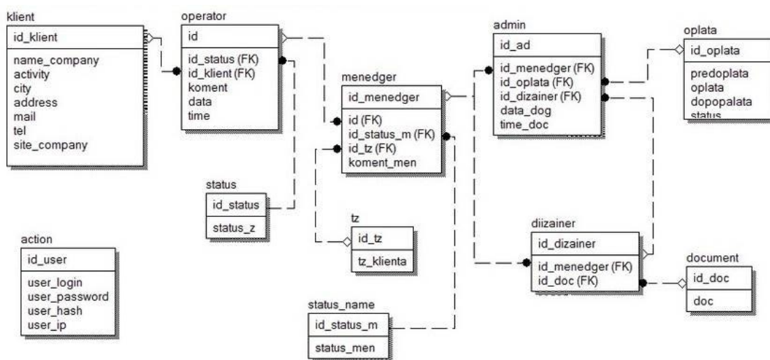
Рисунок 1. Пример логической схемы базы данных
