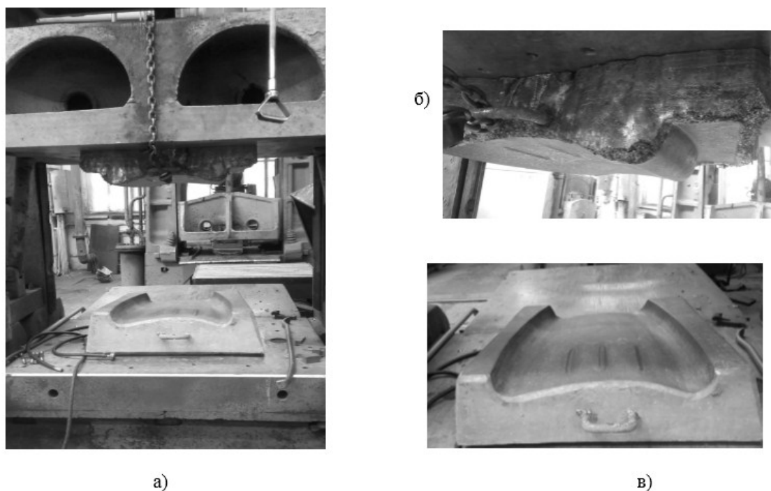
Рисунок 1. а) молот, б) свинцовый пуансон, в) матрица
