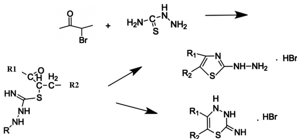
Рисунок 1. Схема взаимодействия 1,3-S,N-нуклеофилов с галогенкарбонильными соединениями
