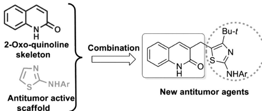
Рисунок 4. Схема синтеза новых противоопухолевых агентов
