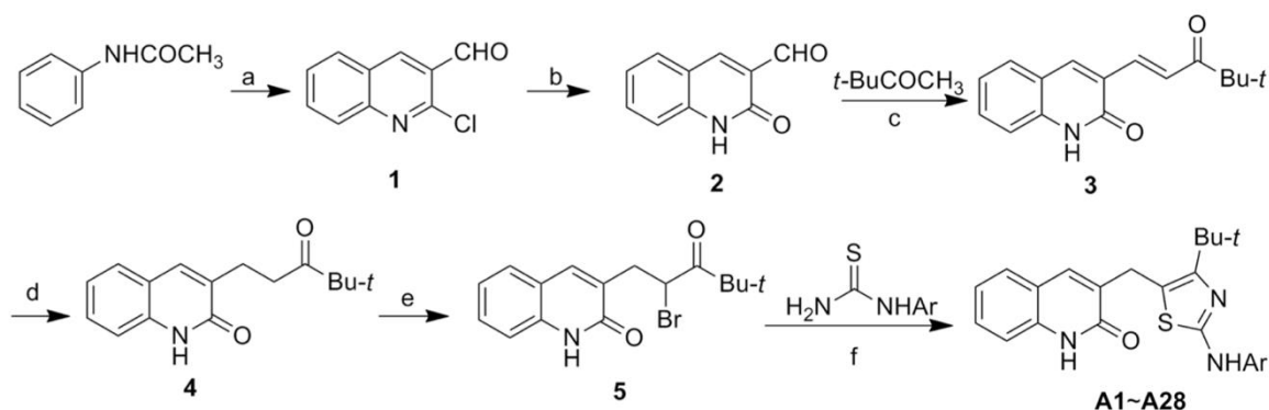
Рисунок 5. Схема синтеза арилтиазольного соединения
