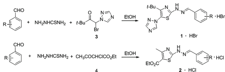
Рисунок 2. Схема синтеза 2-тиазолилгидразона
