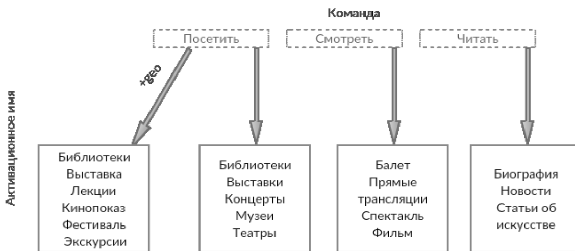
Рисунок 1. Схема навыков
