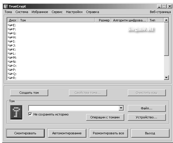
Рисунок 4. Интерфейс TrueCrypt
