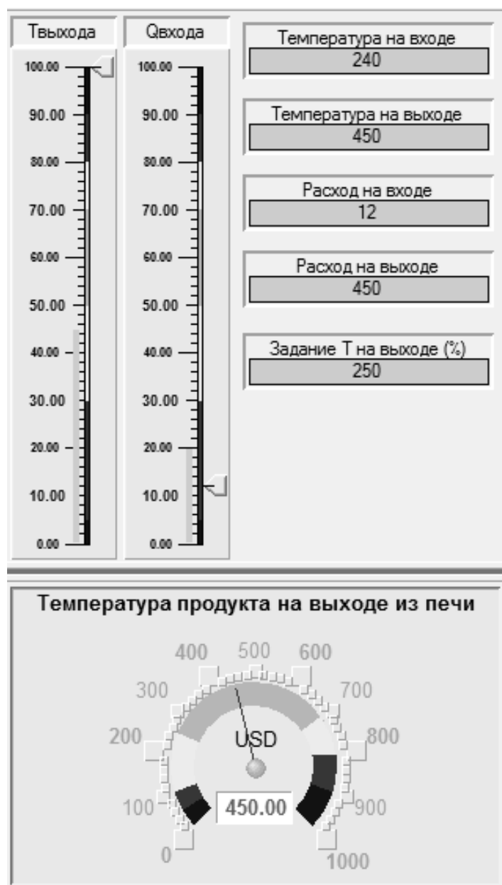
Рисунок 2. Экран значений датчиков
