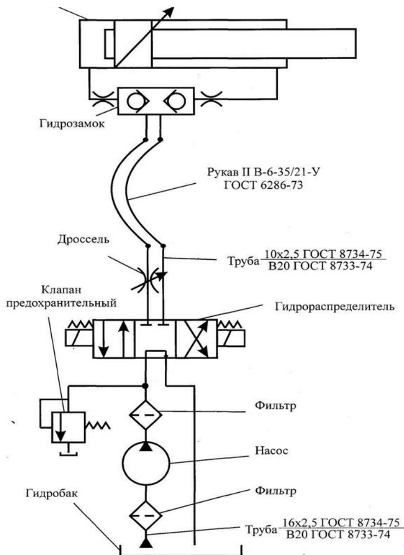
Рисунок 2. Гидравлическая схема управления дозатором
