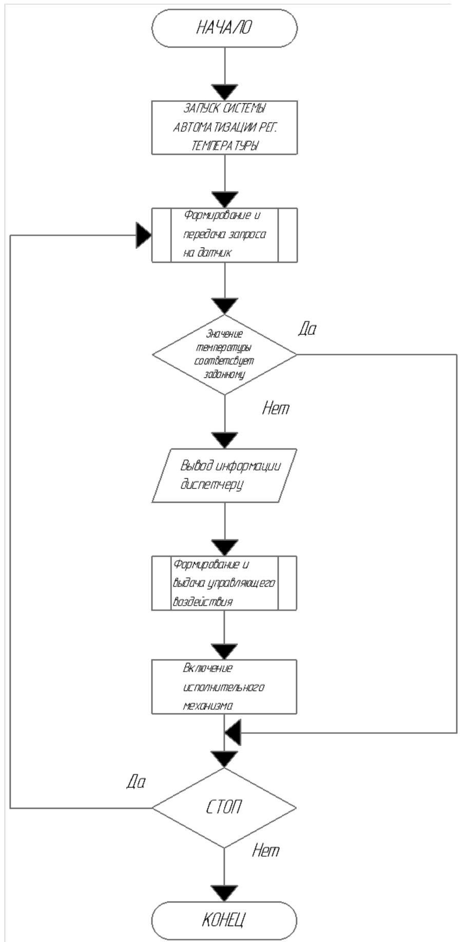
Рисунок 1. Блок-схема алгоритма
