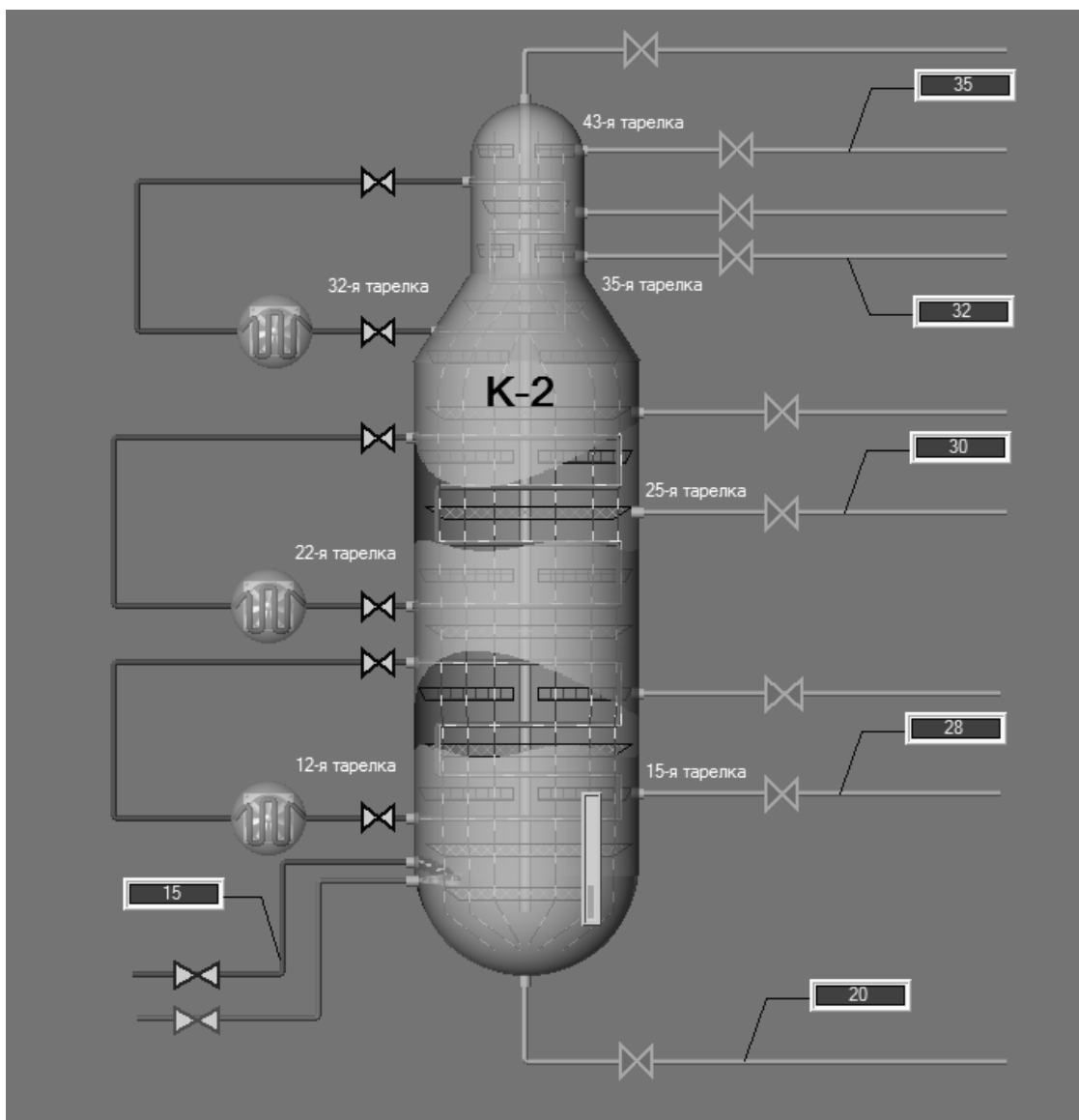
Рисунок 3. Ректификационная колонна
