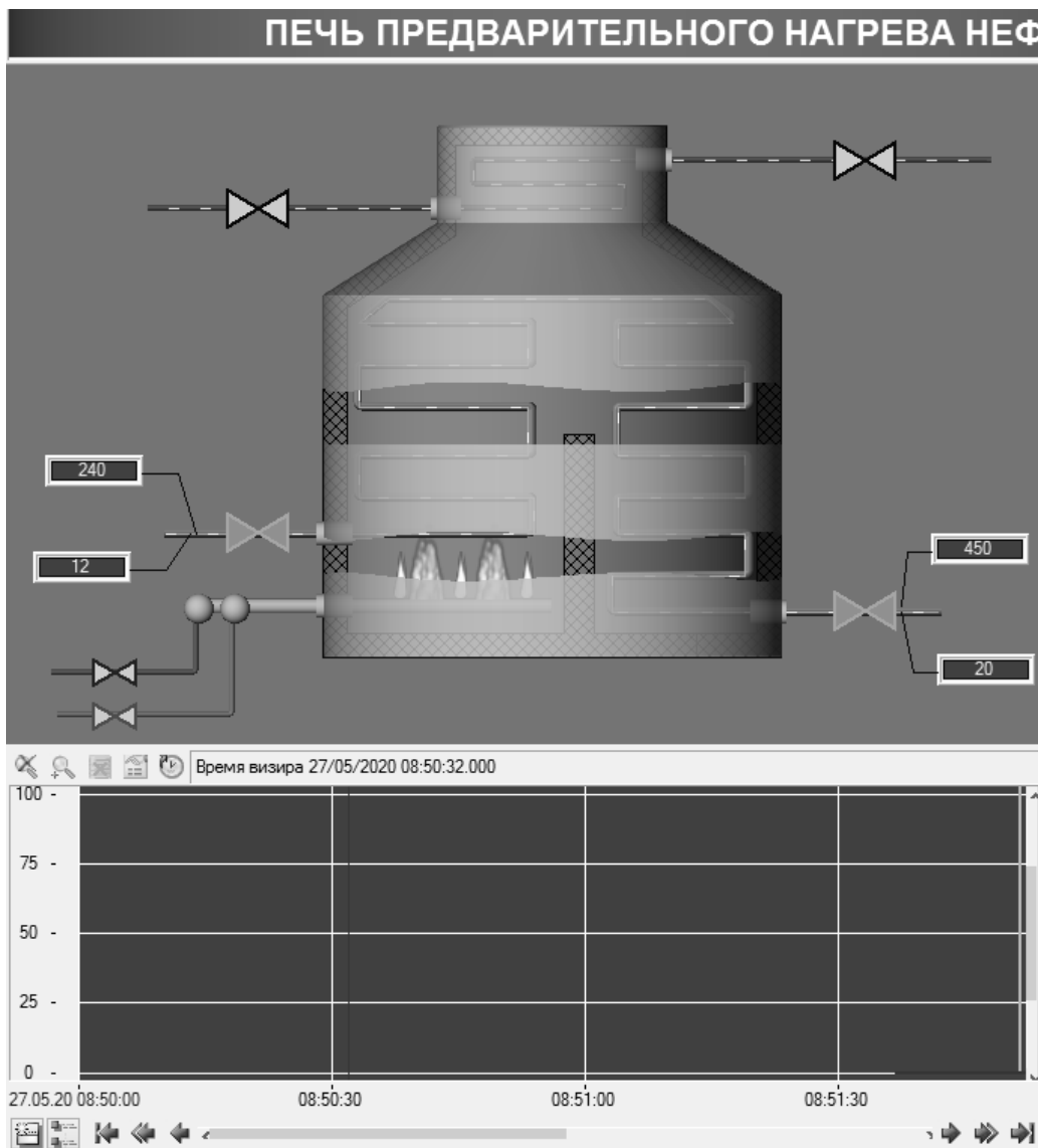
Рисунок 1. Печь предварительного нагрева
