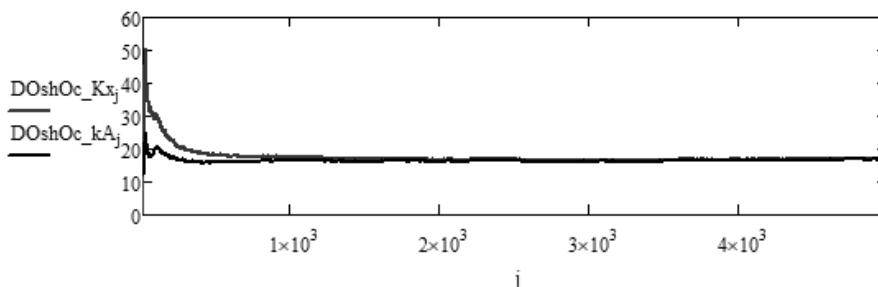
Рисунок 3. Изменение дисперсии ошибок оценок адаптивной финитно-временной фильтрации на текущем интервале времени r-d ( DOshOc\_Kx ) и адаптивного прогноза фильтра Калмана ( DOshOc\_kA ) от дискретного времени i
