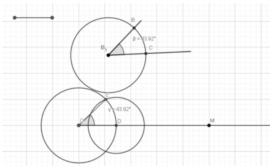
Рисунок 2. Задача на построение циркулем и линейкой
