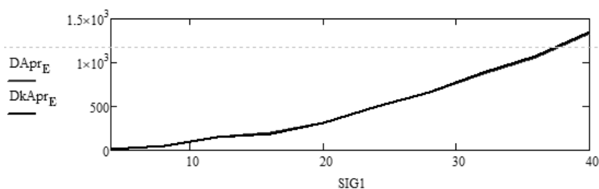
Рисунок 8. Изменение дисперсии ошибки оценки адаптивного финитно-временного прогноза ( D\text{Apr}_E ) и адаптивного прогноза фильтра Калмана ( Dk\text{Apr}_E ) от изменения параметра SIG1
