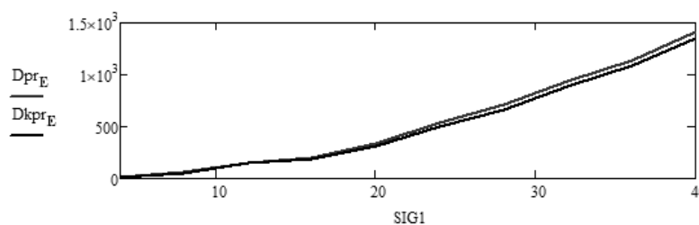
Рисунок 7. Изменение дисперсии ошибки оценки финитно-временного прогноза ( Dpr_E ) и прогноза фильтра Калмана ( Dkpr_E ) от изменения параметра SIG1
