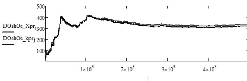
Рисунок 2. Изменение дисперсии ошибок оценок финитно-временного прогноза на текущем интервале времени r-d ( DOshOc\_Xpr ) и прогноза фильтра Калмана ( DOshOc\_kpr ) от дискретного времени i
