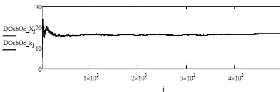
Рисунок 1. Изменение дисперсии ошибок оценок финитно-временной фильтрации на текущем интервале времени r-d ( DOshOc\_X ) и фильтра Калмана ( DOshOc\_k ) от дискретного времени i
