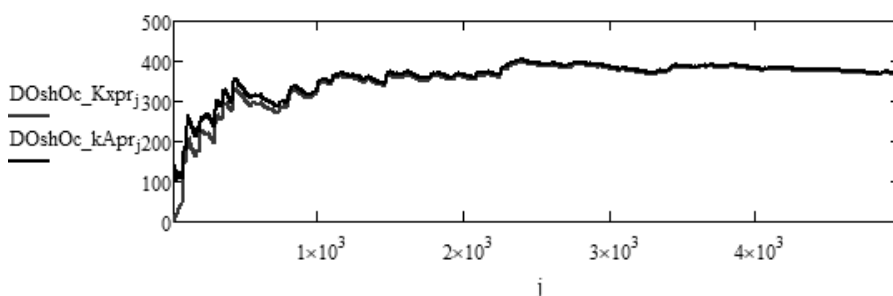
Рисунок 4. Изменение дисперсии ошибок оценок адаптивного финитно-временного прогноза на текущем интервале времени r-d ( DOshOc\_Kxpr ) и адаптивного прогноза фильтра Калмана ( DOshOc\_kApr ) от дискретного времени i
