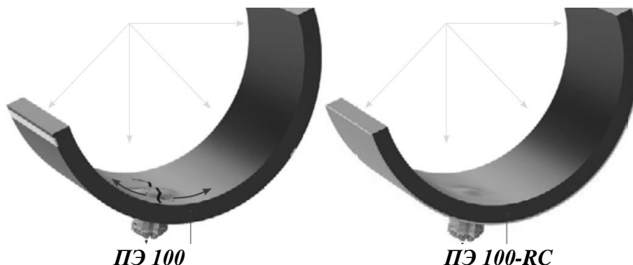
Сурет 2. Полиэтиленнің әр түрлі маркаларына нүктелік жүктеменің әсері
