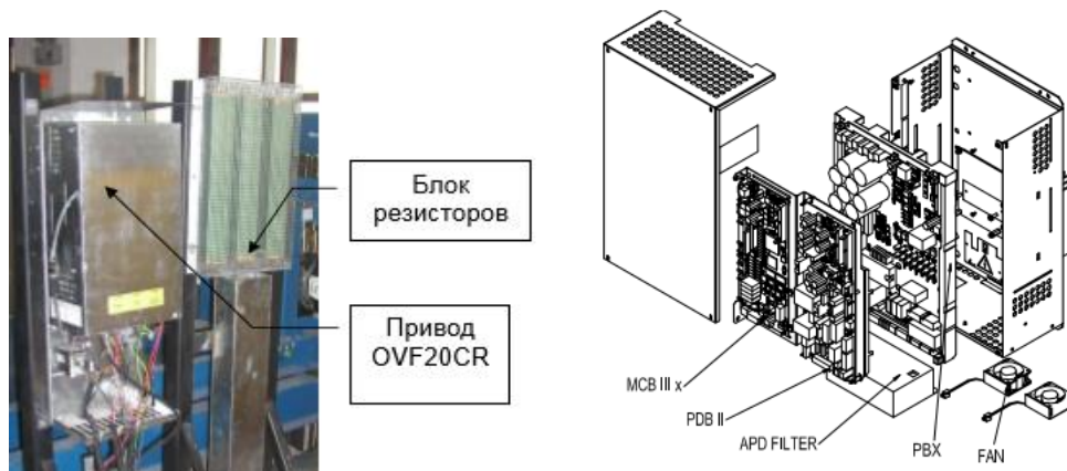
Рисунок 1. Общий вид преобразователя частоты
