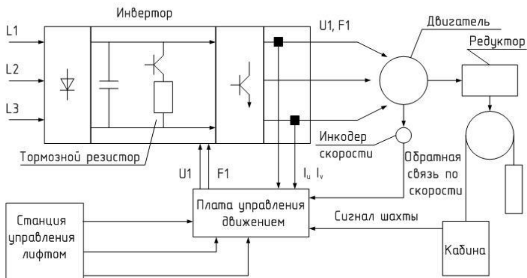
Рисунок 2. Схема управления
