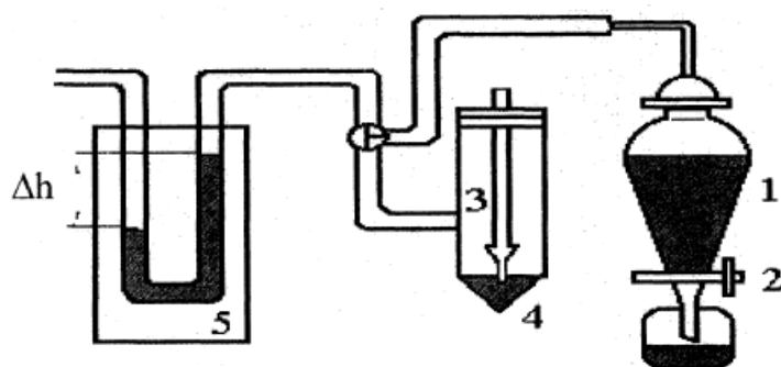
Рисунок 1. Схема установки для измерения поверхностного натяжения жидкости (прибор Ребиндера):
