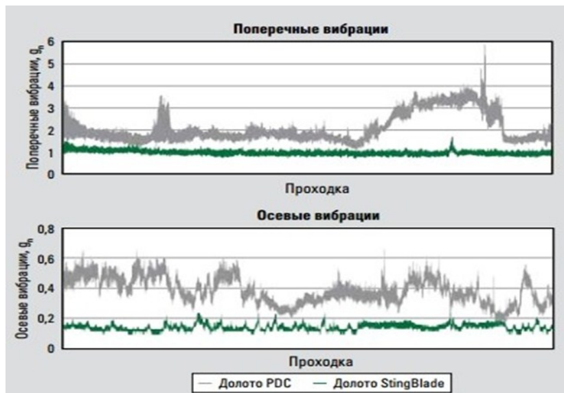
Рисунок 4. Диаграмма вибрационной устойчивости
