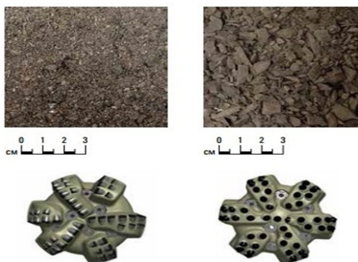
Рисунок 5. Фрагменты шлама
