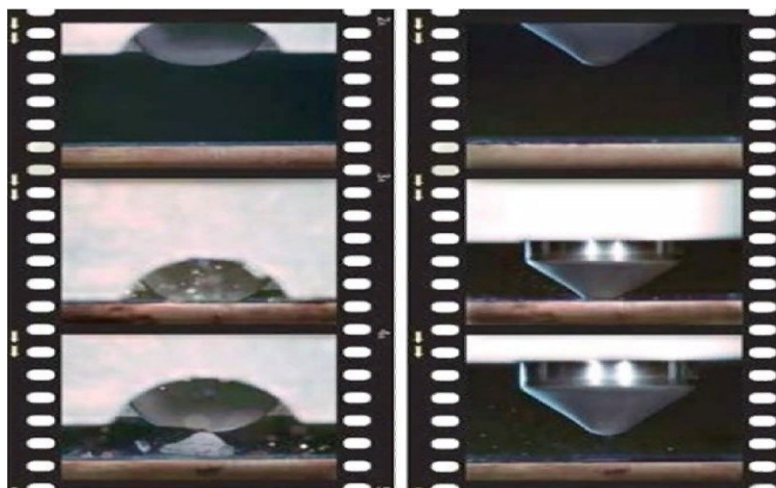
Рисунок 3. Испытания износостойкости долот
